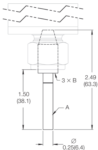
튜브 스테브
