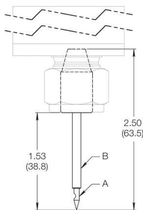
동심(Concentric) 니들
