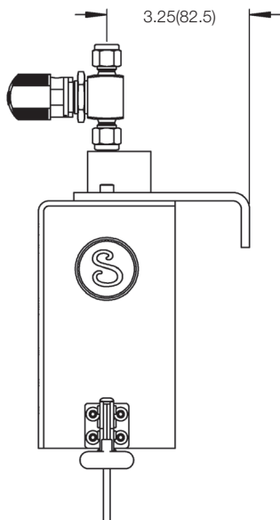
측면도 - 직선형
