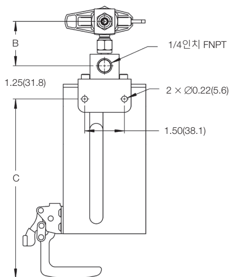
후면도 - 직각형
