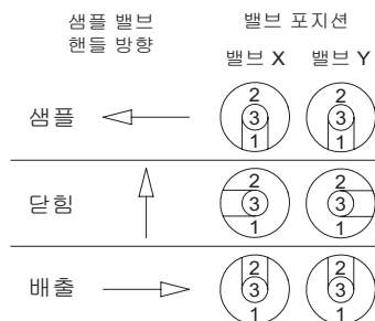
2-밸브 방향 전환형 밸브
