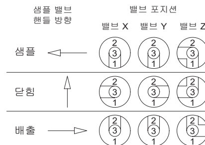
3-밸브 방향 전환형 밸브
