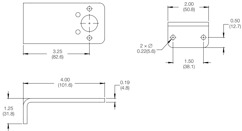
벽면 브라켓 (주문 번호 - 304-GSV-MBK-M)
