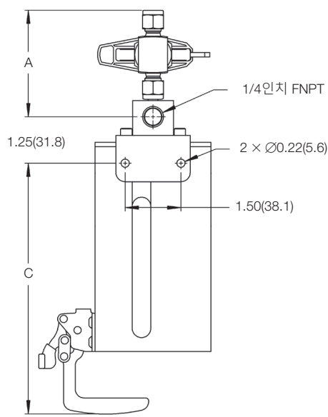
후면도 - 직선형
