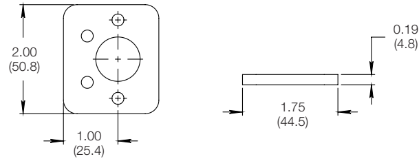
덮개/인클로저 어댑터 (주문 번호 - 304-GSV-MBK-S)
