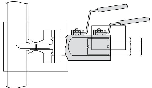
Vanne d'injection avec clapet anti-retour intégré et raccordement NPT
