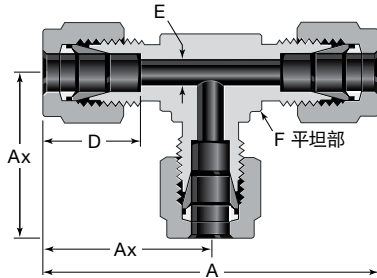
卡套管孔口完全相同。
