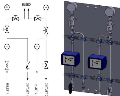
API 682 PLAN 54
