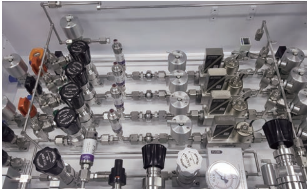
반도체 Gas module
