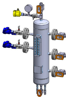
API 682 Plan 53A
