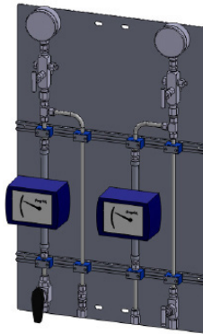
API 682 Plan 54
