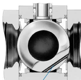
Externe Belüftungsoption
