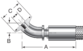
새니터리 퀵클램프 45° 엘보우
