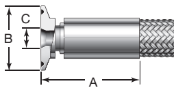
JIS(A)/ISO 2852-타입 새니터리①
