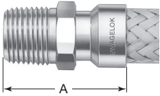
수동 용접 스타일— 1 in. 초과
