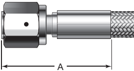
암나사형 VCR 금속 가스켓 양면 접속 피팅
