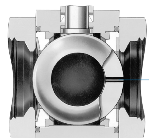
Interne Belüftungsoption
