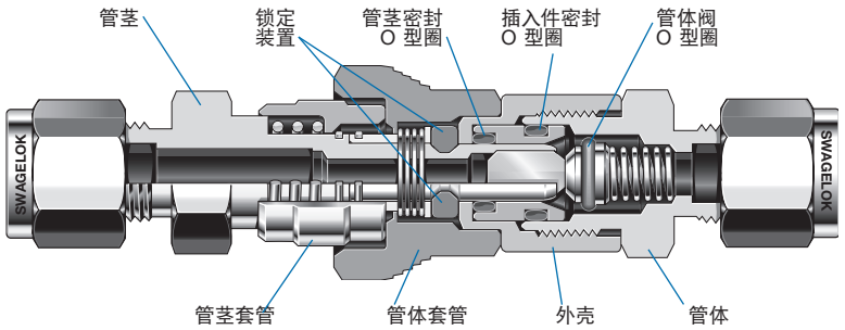
单端关断 (SES0)
