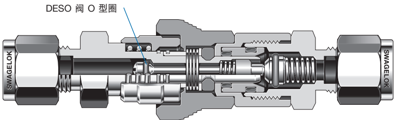
双端关断 (DESO)—红色管茎套管
